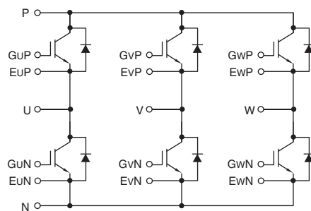
CM200TU-5F
