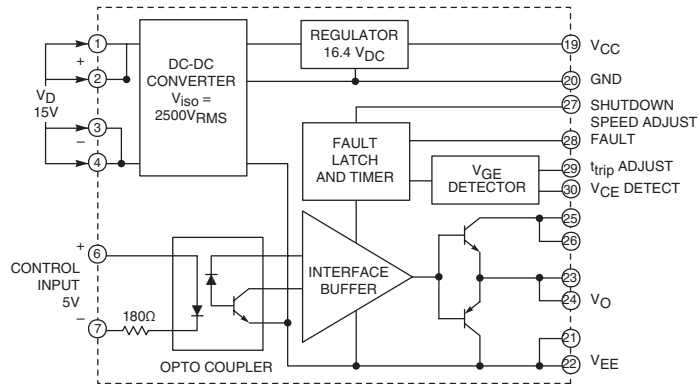
VLA500-01, VLA500K-01R
