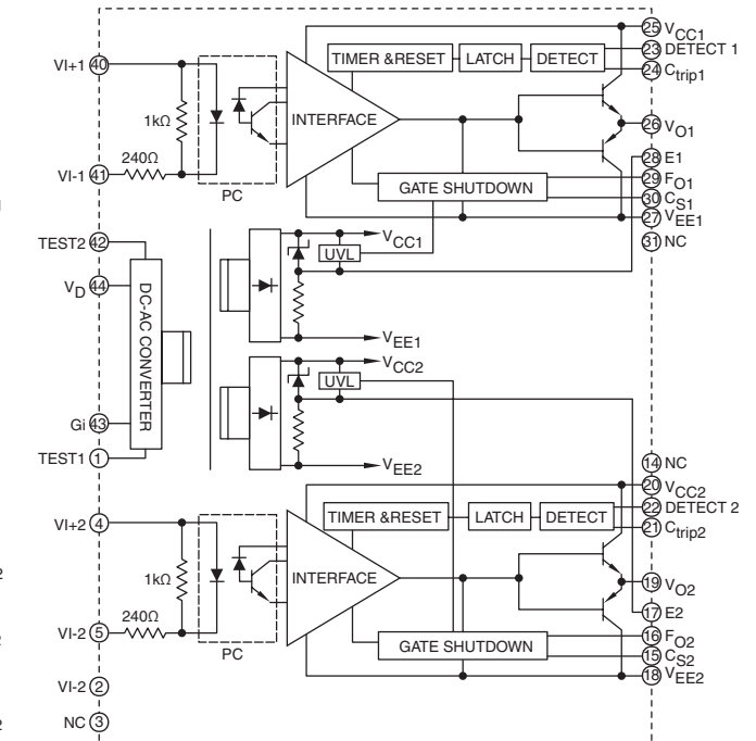
VLA567-01R
