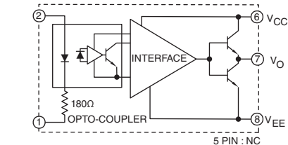
VLA507-01, VLA513-01
