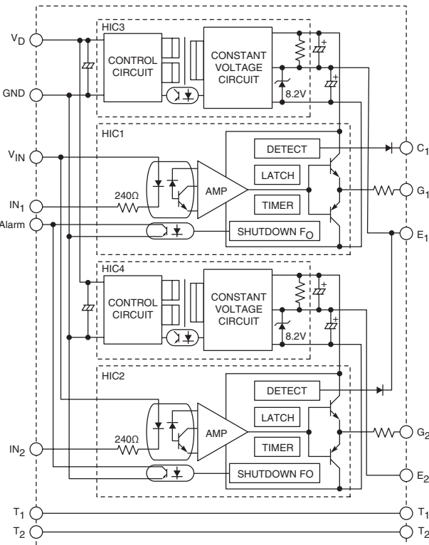
VLA536-01R
