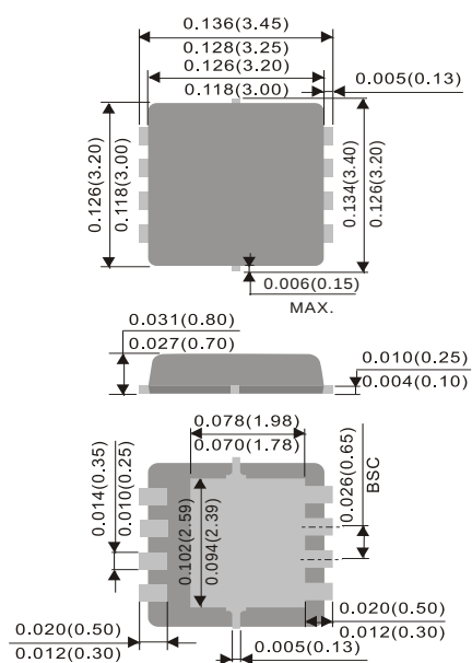
DFN3333-8L Dimension
