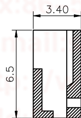
SECTION D-D
